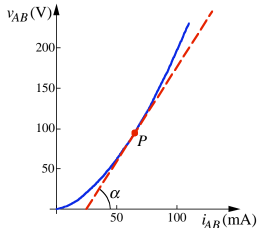
Fig. 4.- Gráfica v_{AB}(i_{AB}) de una lámpara de incandescencia y tangente en un punto P de la curva.
