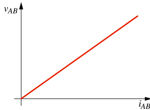
Fig. 3.- Representación gráfica de la relación tensión-intensidad de una resistencia R_{AB} .
