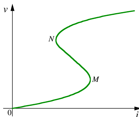
Fig. 5.- En esta gráfica la resistencia dinámica es negativa desde M a N.
